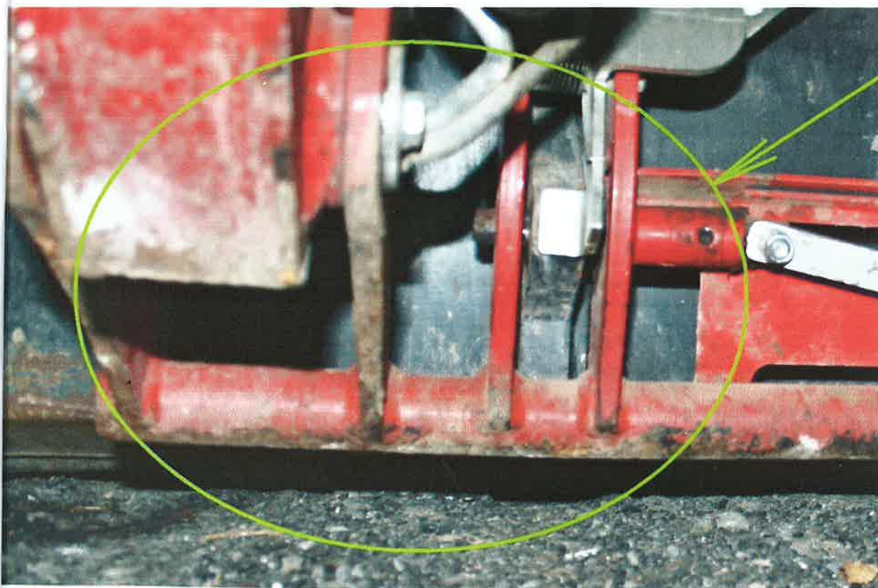
6. Detailní pohled na spodni trubku nosniku s čepy pro ovládací prvky, kdy trubka je vyhnutá, čepy vyosené..jpg 09.07.2020 13:19
